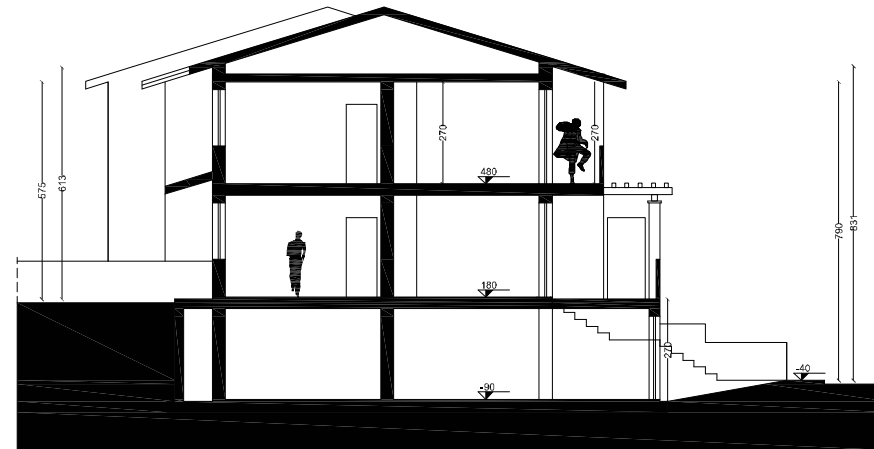
SEZIONE C-C
